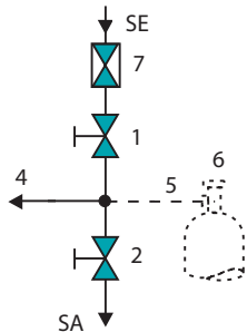
DPB 502 (2-Port-Version)
