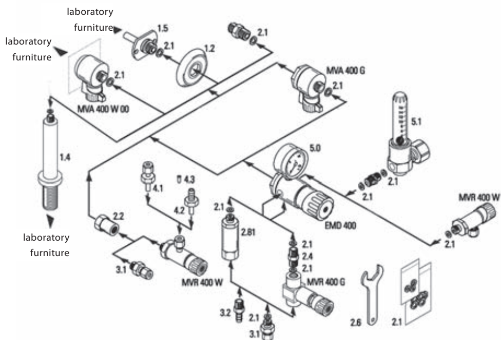
EMD 400-01
