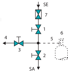
DPB 503 (3-Port-Version)
